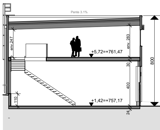
Coupe 1:200
