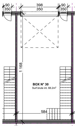
Rez-de-chaussée 1:200
